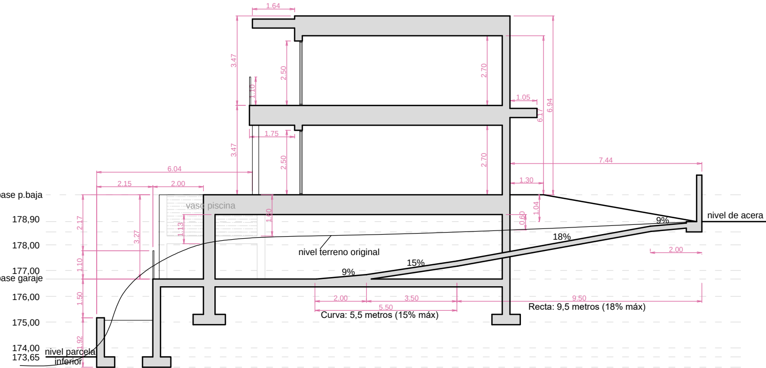
SECCIÓN - ESQUEMA DE ALTURAS E: 1/150
