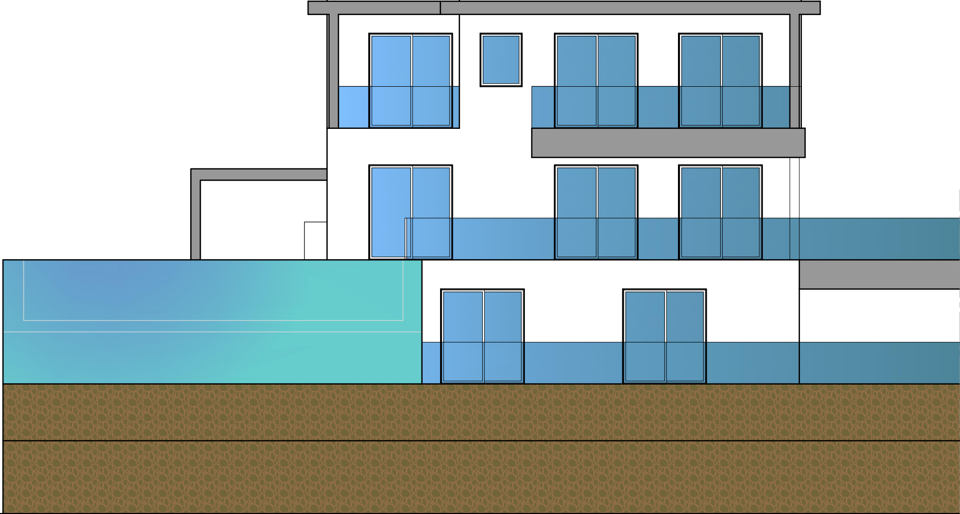
ALZADO SUR (VIVIENDA VIENA Nº 6)
