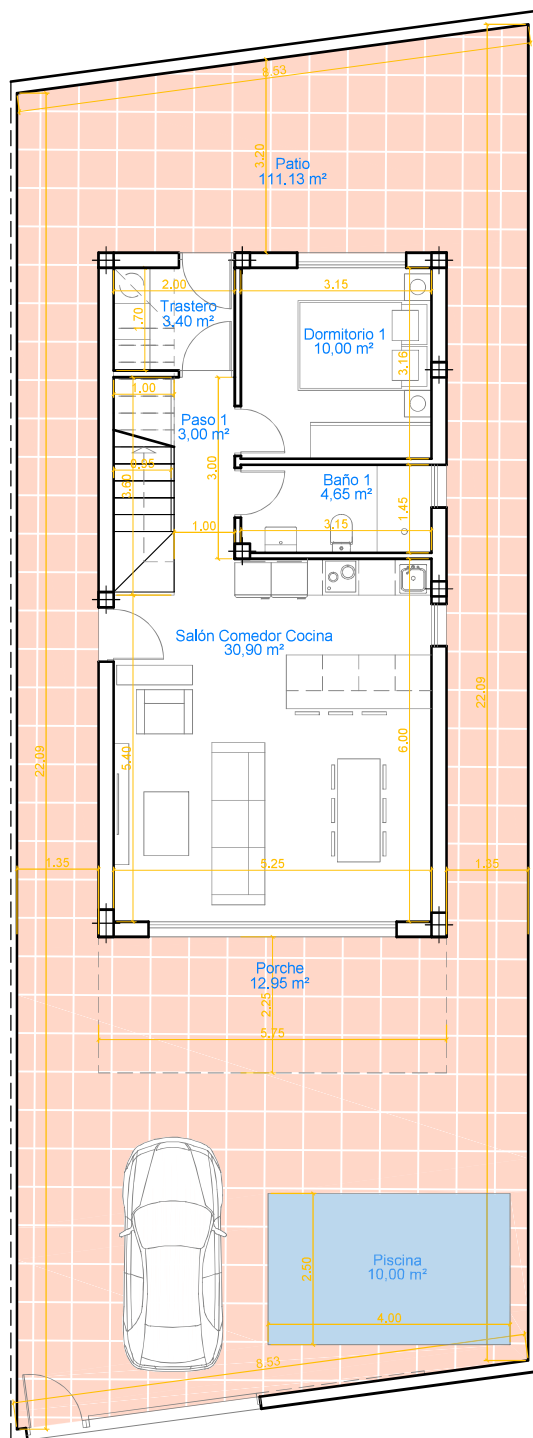
Planta Baja
