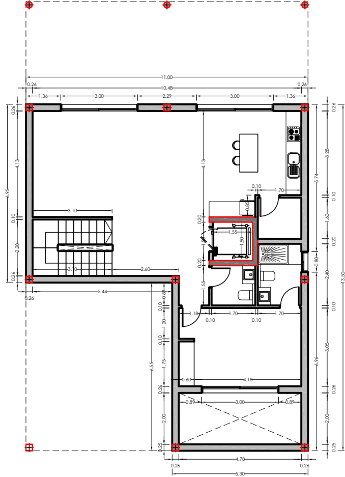
PLANTA -1
