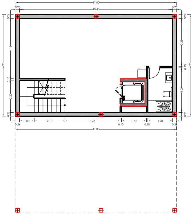
PLANTA SÓTANO
