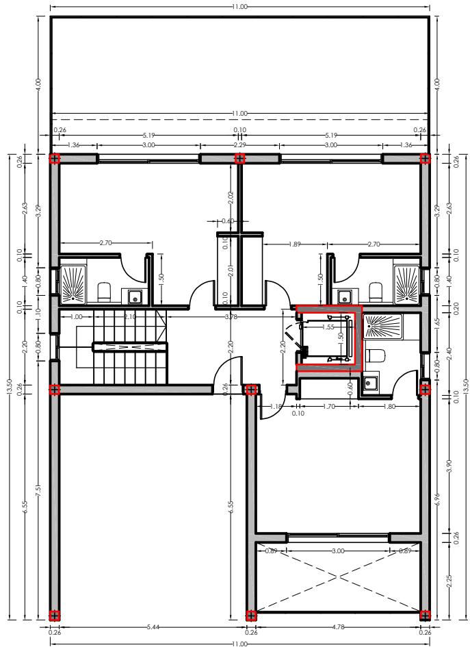
PLANTA 0
