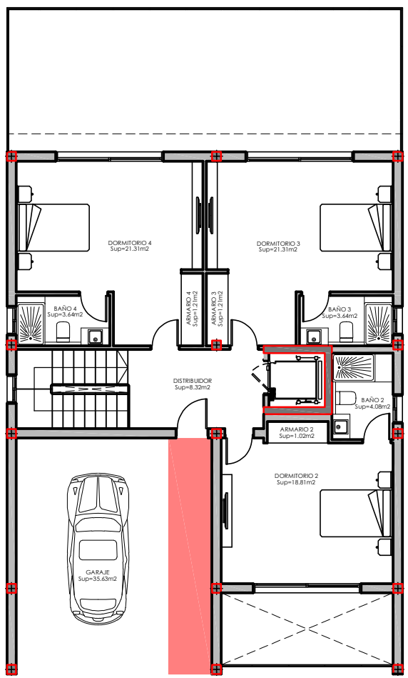
PLANTA 0 SUP: 148.16 m2
