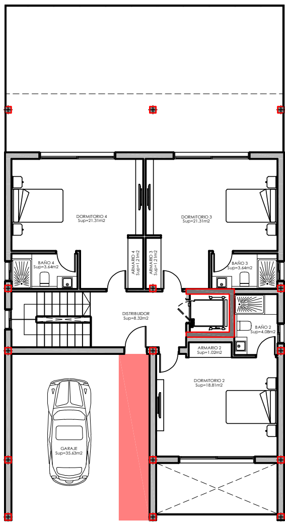
PLANTA 0 SUP: 148.16 m2
