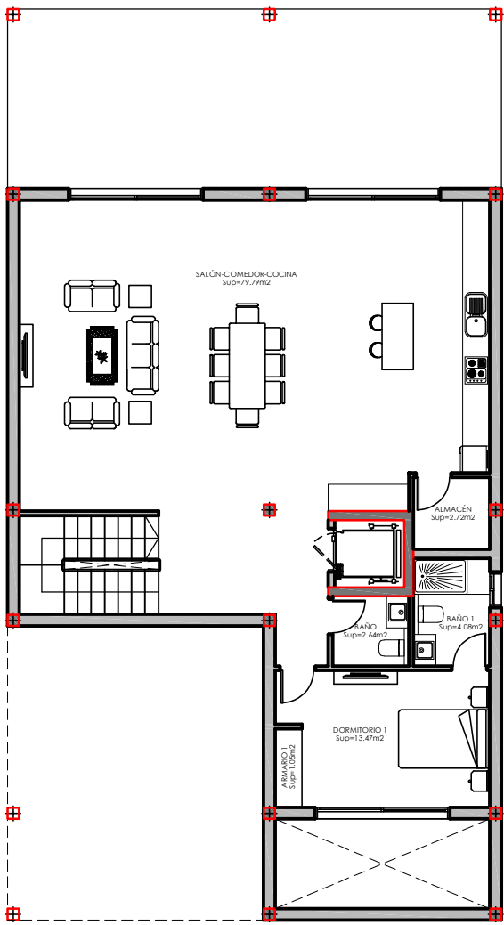
PLANTA -1 SUP: 130.04 m2
