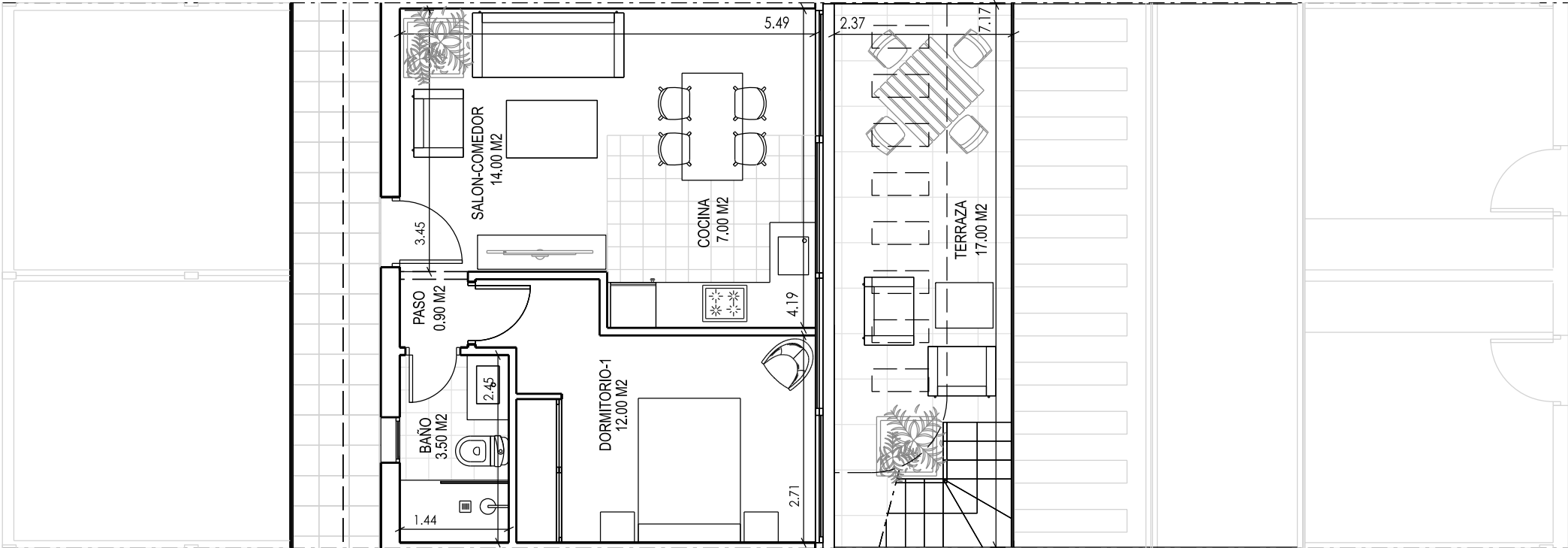
PLANTA SEGUNDA
