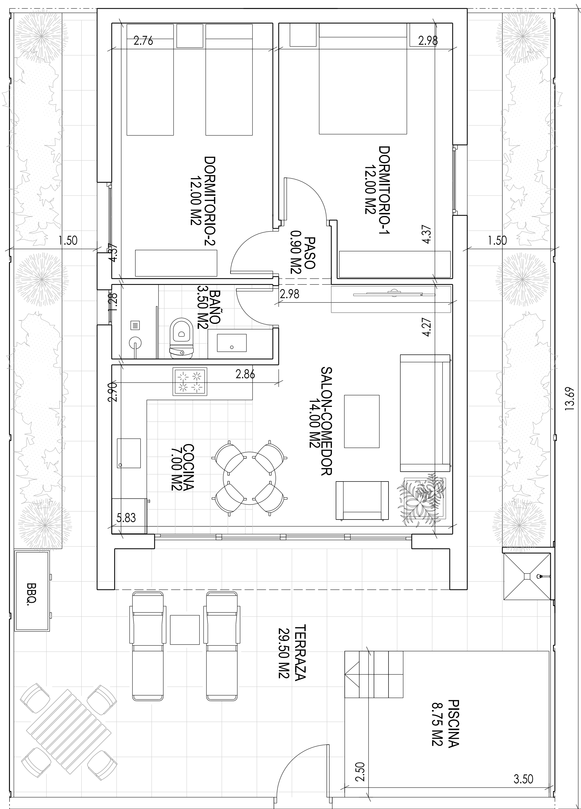
PLANTA BAJA
